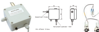
Kabelbrücke
